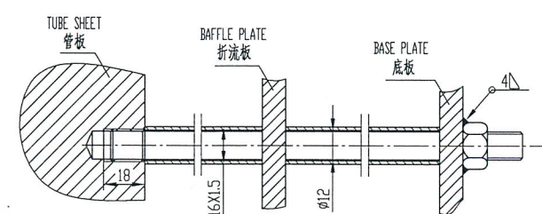
TIE ROD DRAWING 拉杆结构图
